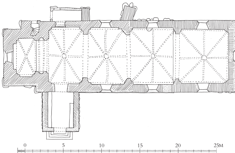
Fig. 8. Grundplan. 1:300. Målt af H. P. Knudsen 1963, suppleret og tegnet af Pia K. Lindholt 2024. Signaturforklaring s. 9. – Plan. Key on p. 17.
