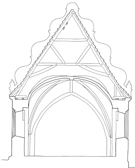
Fig. 7. Tværnsnit. 1:150. Målt og tegnet af Pia K. Lindholt 2024. – Cross-section.
